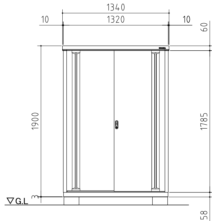
正面図
